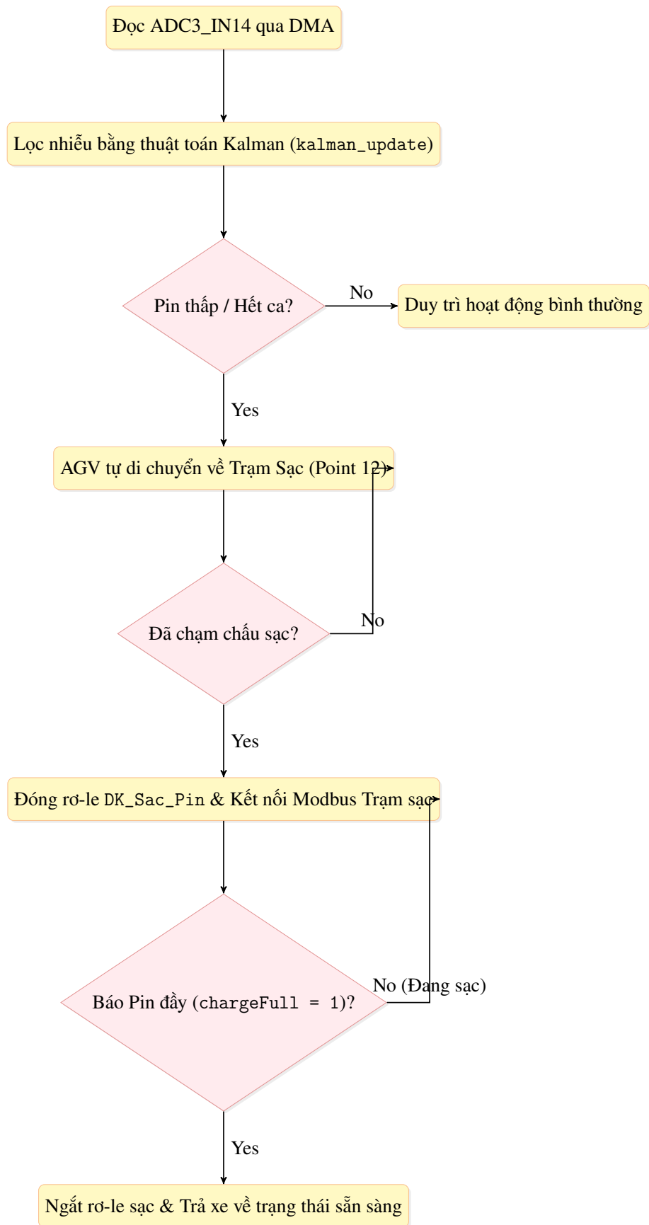
Hình 4.6 Sơ đồ luồng đo điện áp pin Kalman và chu trình sạc tự động.
